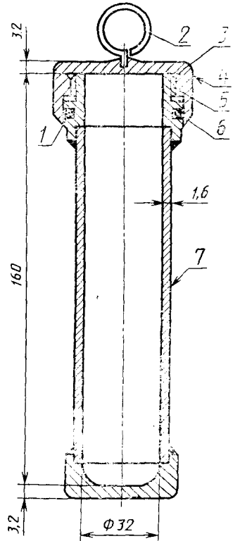
Испытательная бомба
